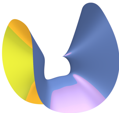
abstrakte Welt
